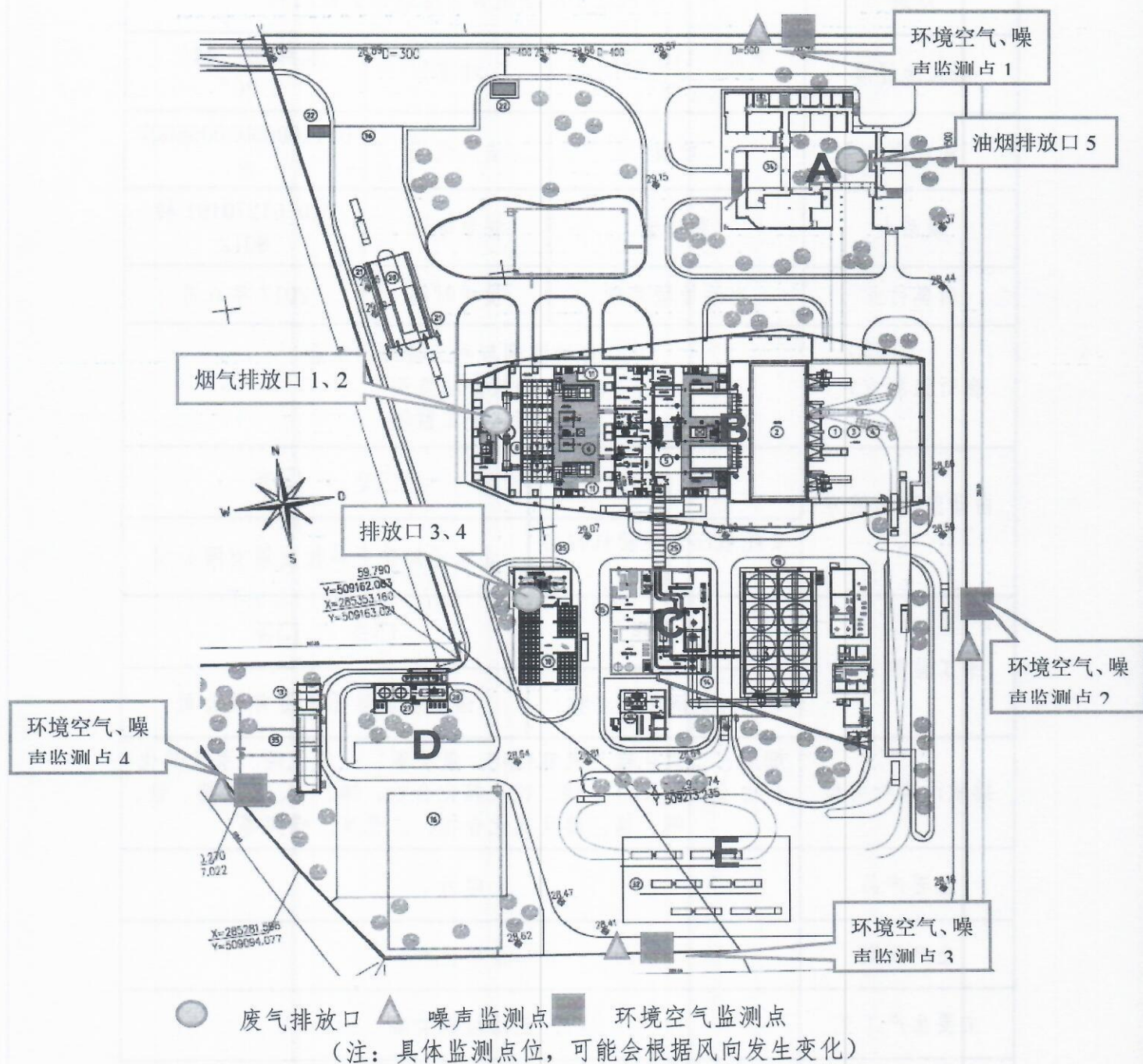
图 2: 南宫生活垃圾焚烧厂厂区平面图及监测点位置图
